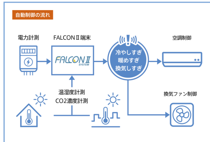
▲温湿度・CO2 濃度の計測から、空調・換気扇の移動制御の流れ
